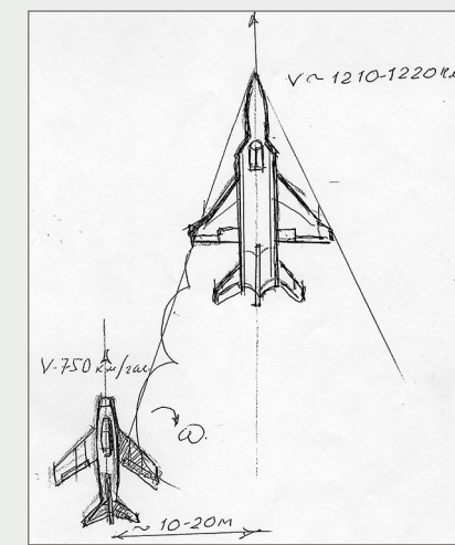
Реконструкция катастрофы МиГ-15УТИ в рисунках А.А. Леонова
